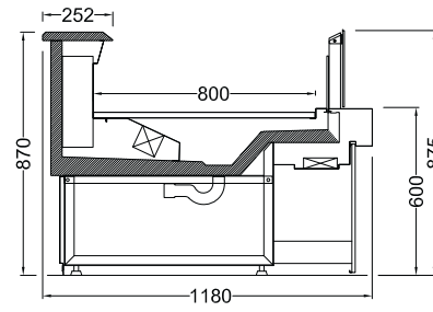
NEVA 112-DÜZ-S
