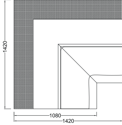
NEVA 102-DÜZ-DK
