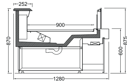
NEVA 122-DÜZ-S
