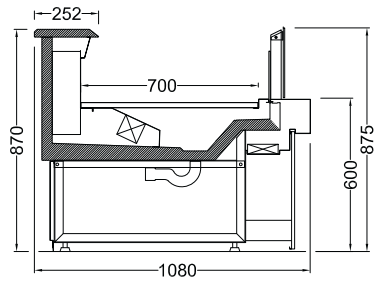
NEVA 102-DÜZ-S
